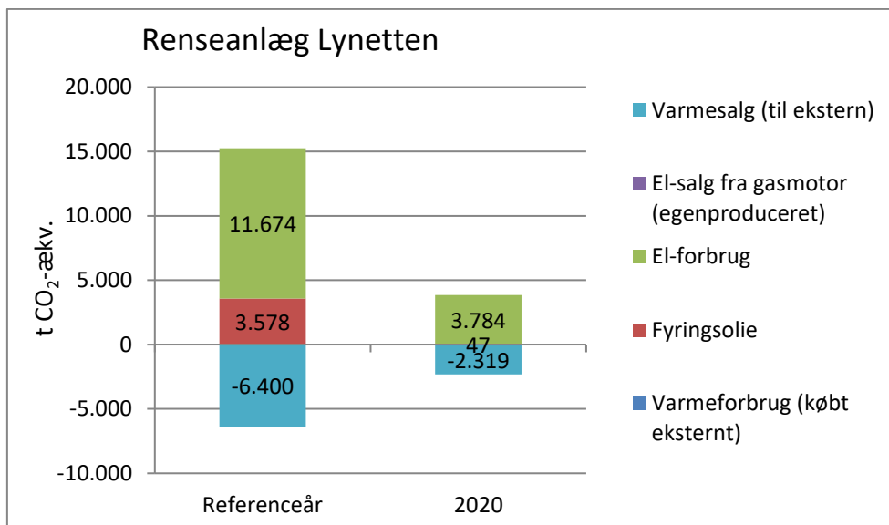
Figur 5: Fordeling af energiforbrug og energiproduktion fordelt på energiformer på Renseanlæg Lynetten
