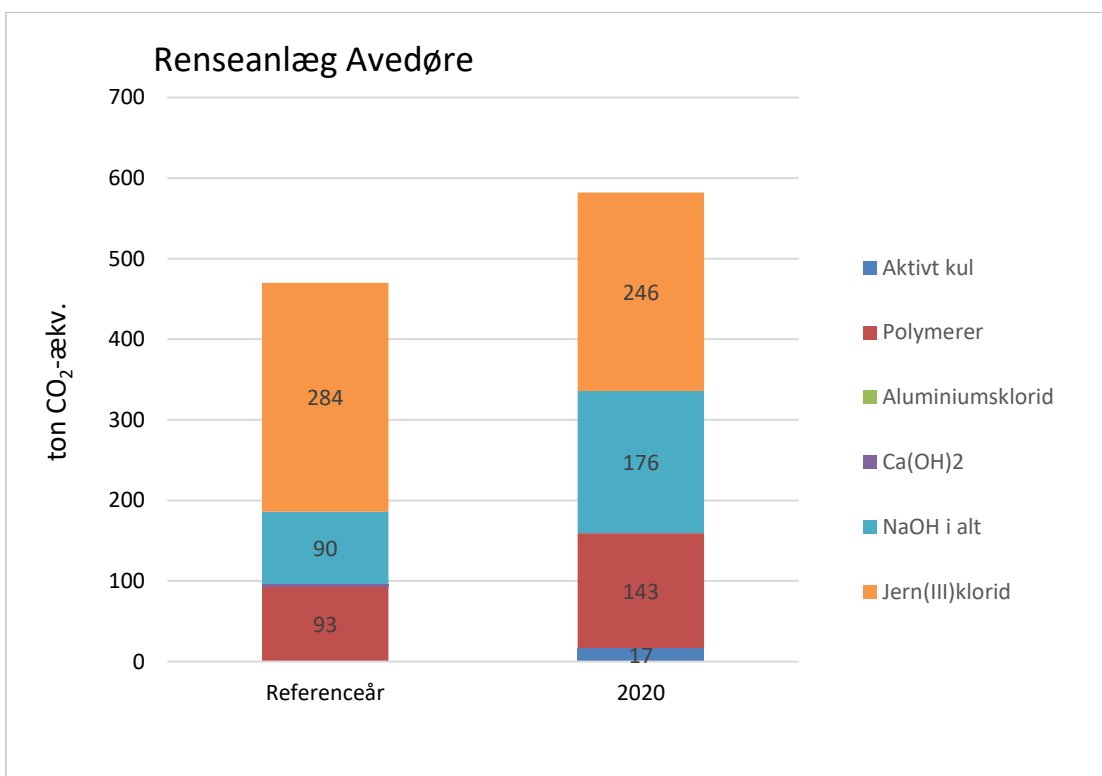
Figur 8: Ressourceforbrugets CO 2 -bidrag, opdelt på underkategorier for Renseanlæg Avedøre
